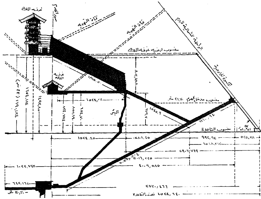
الأبعاد الداخلية للهرم الأكبر موضحة بالبوحة الهرمية (وحدة القياس الرمي) للثبوت التي يعبر الخط البياني الذي تتركه الممرات والطرق .....
