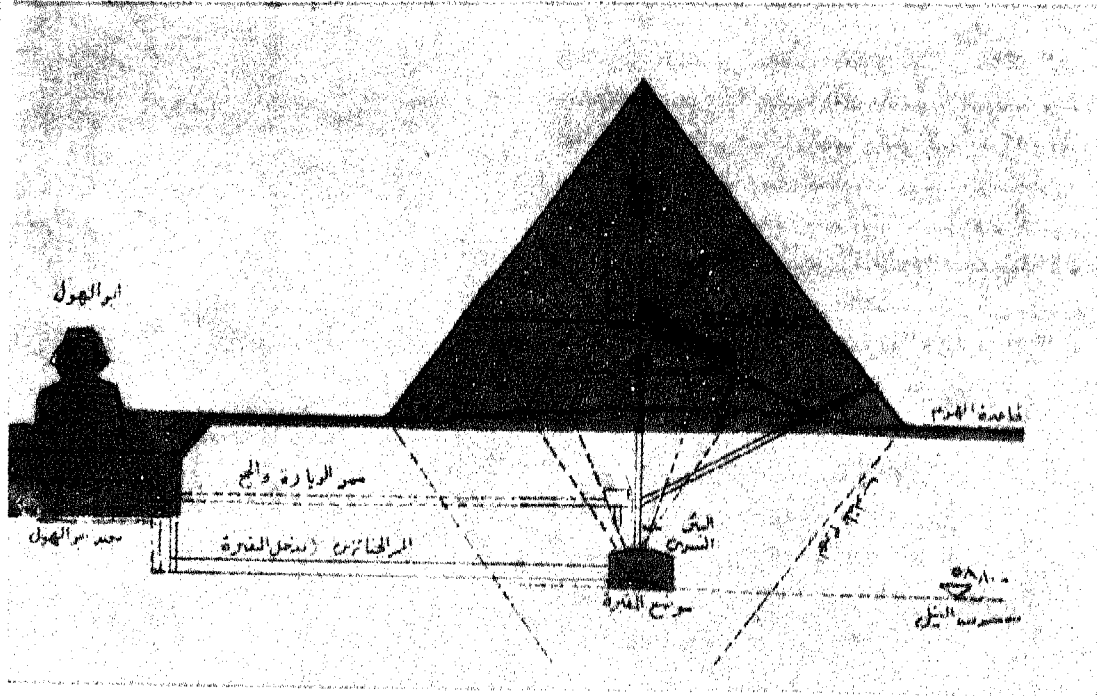
موضع المقبرة ومدخلها بالنسبة لمحور الهرم وقاعدته وغرفة الروح والبئر السرى وقاعة أبو الهول ونظريات المؤرخين
