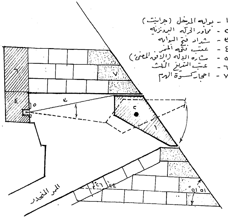
قطاع خيال مدخل الهرم وبوابته الأصلية محورية الحركة (أبحاث أندريه بوشان)
