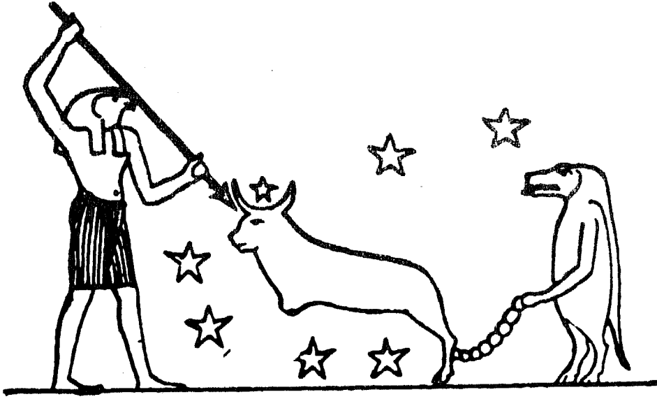
مجموعه الدب الأكبر
